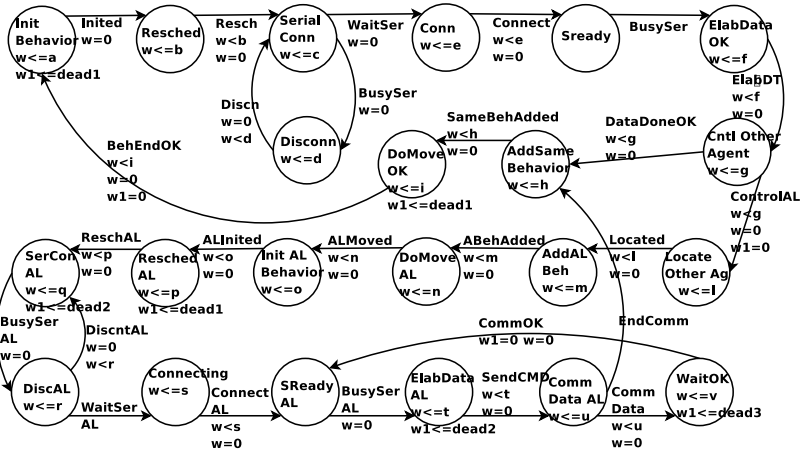
Fig. 4. Nimrod TA
