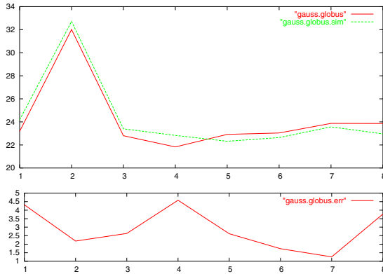
Fig. 5. Gauss-Siedel Simulation
