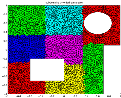
Fig. 1. Test Grid
